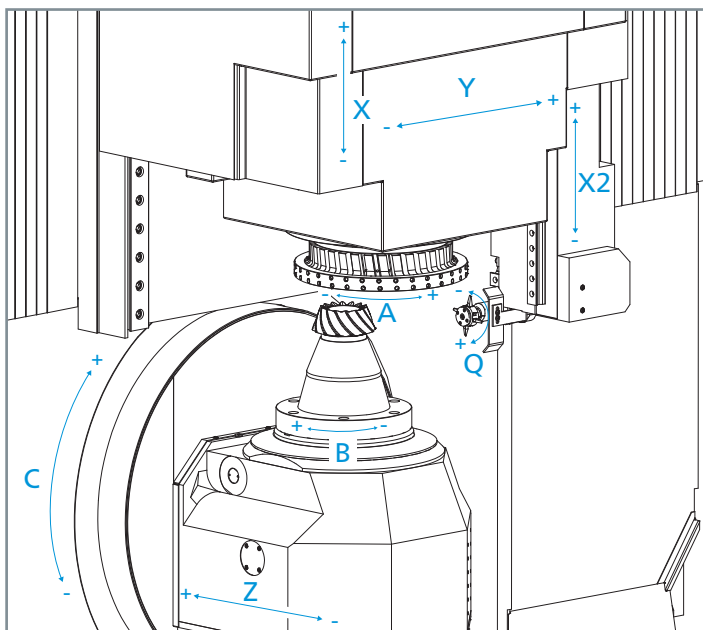
Achsanordnung einer Oerlikon Kegelrad-Fräsmaschine C 50
