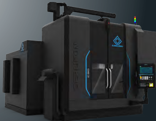
Oerlikon Kegelrad-Fräsmaschine C 50, kundenspezifische Variante mit zahlreichen Ausstattungsdetails
